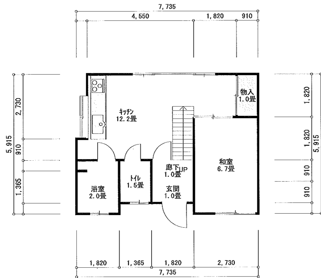
1階 縮尺 1/100
