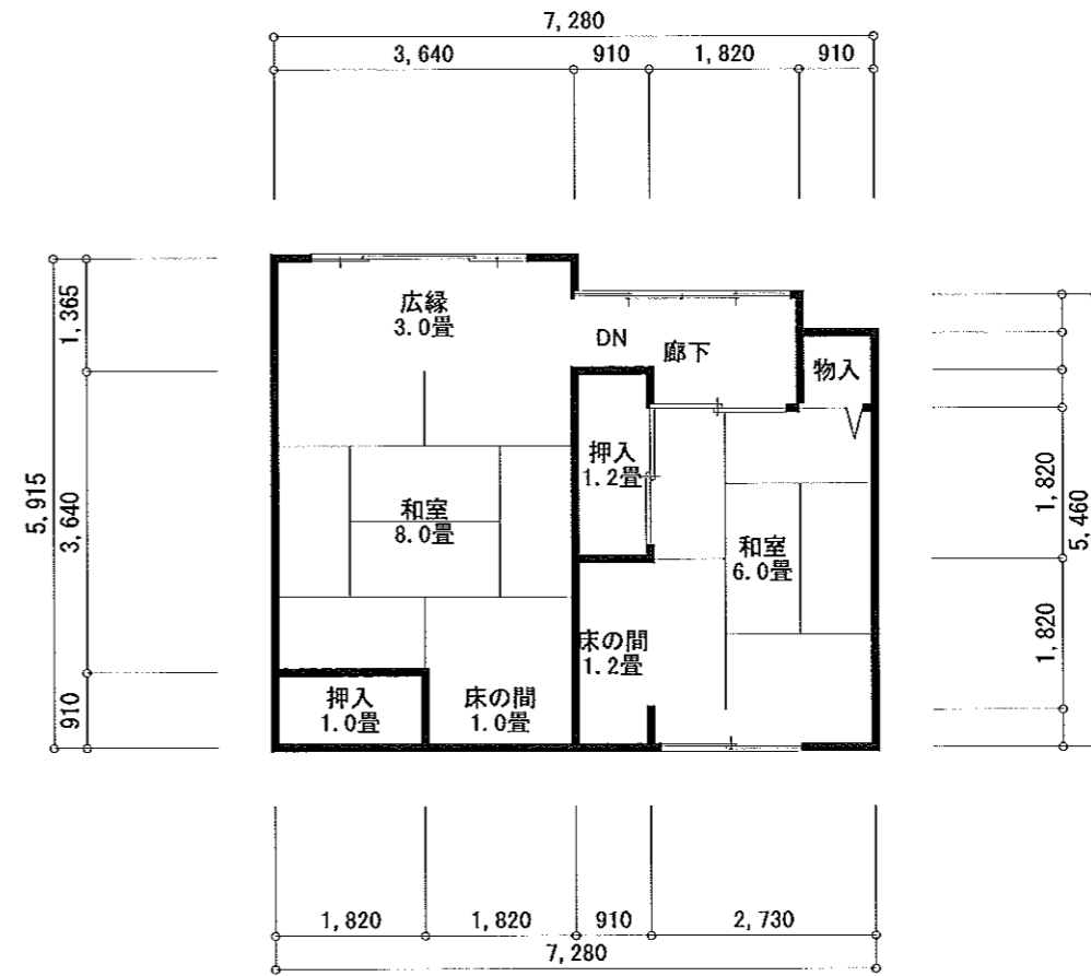
2階 縮尺 1/100
