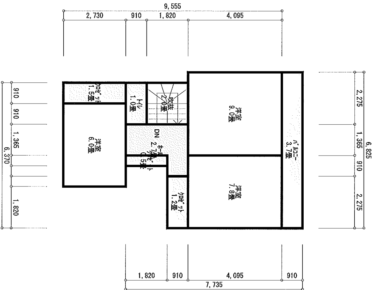
2階 縮尺 1/100
