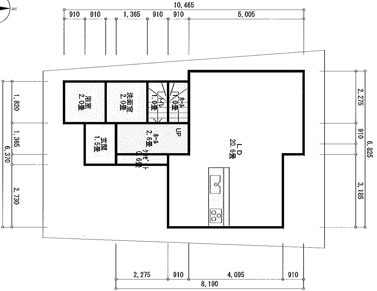
1階 縮尺 1/100
